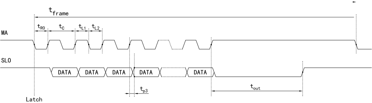
图5 SSI 时序图
