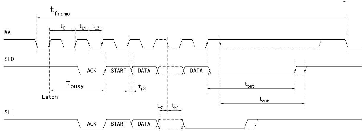
图2 BISS_C 时序图
