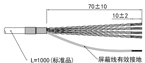
电缆连接
